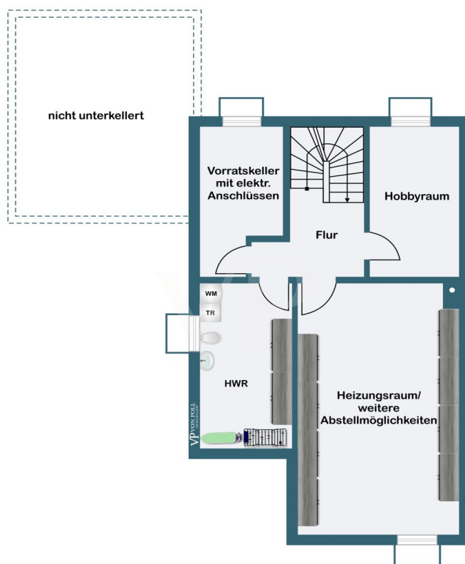
Kellergeschoss
