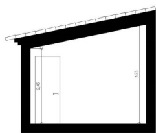
SECCION B-B
