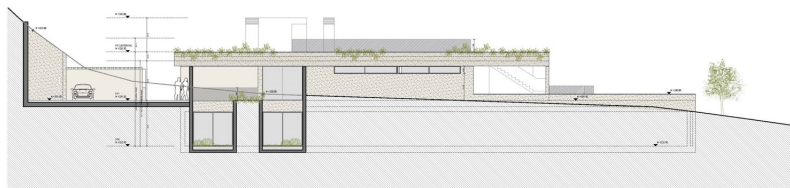
ALZADO 02 - FACHADA SUROESTE # 1/100-043
