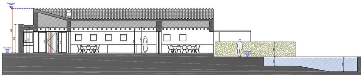
SECCIÓN 1 E: 1/150
