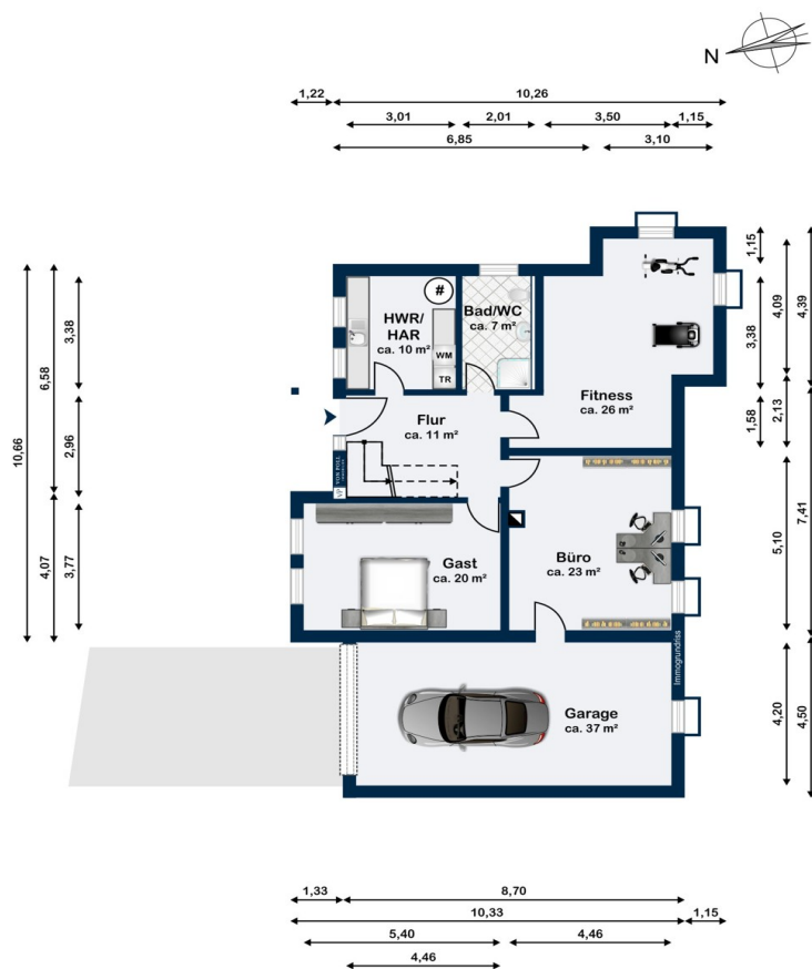
Kellergeschoss
