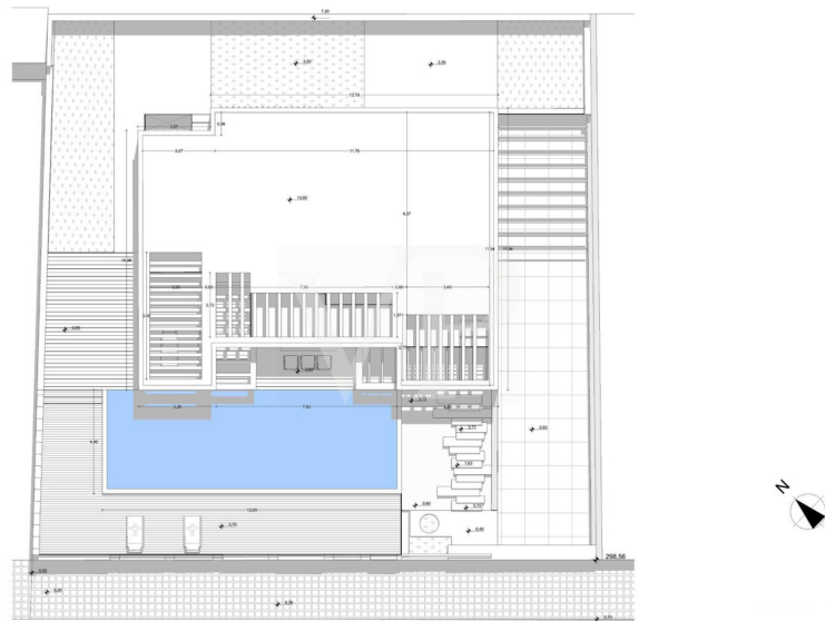
PLANTA DE TECHO 1:50
