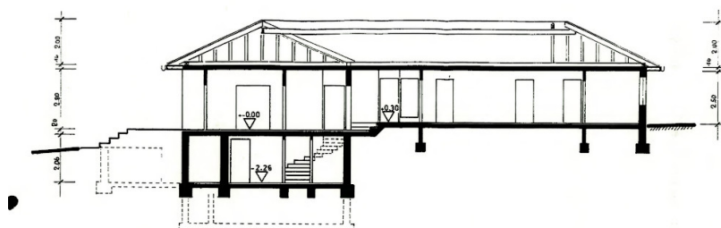
SCHNITT B-B
