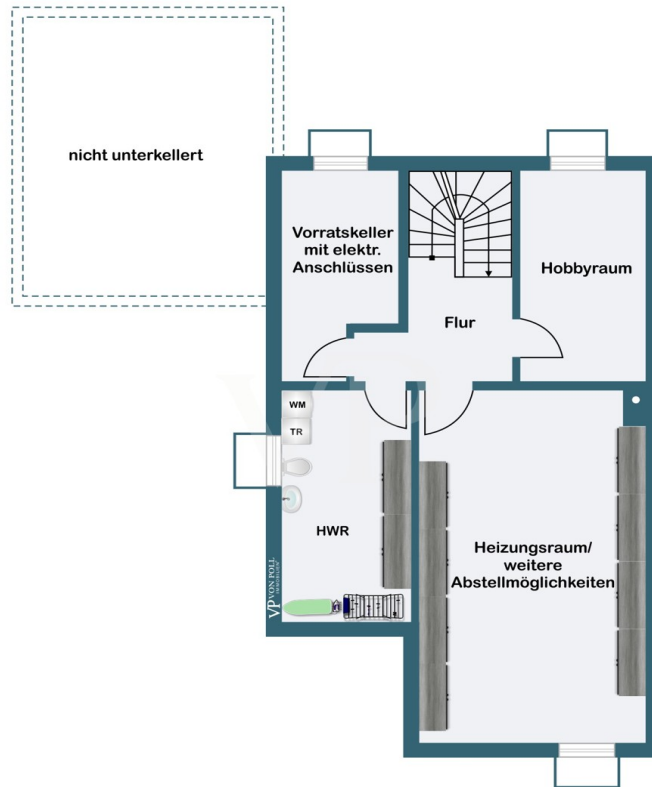
Kellergeschoss
