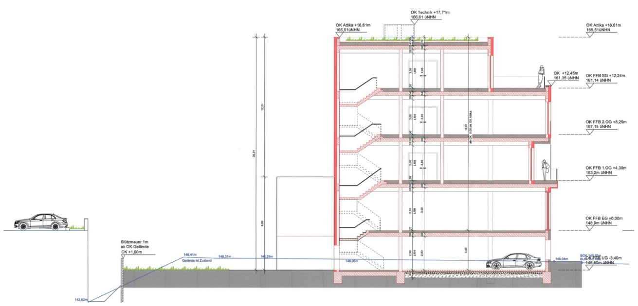
Schnitt B-B
