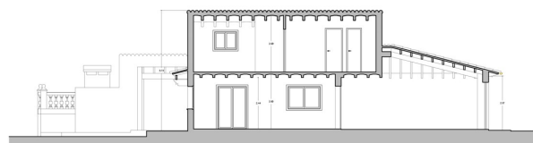
SECCIÓN S-02
