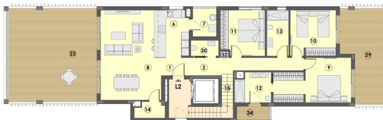
PLANTA SEGUNDA
