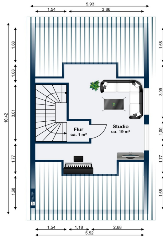
Dachgeschoss
