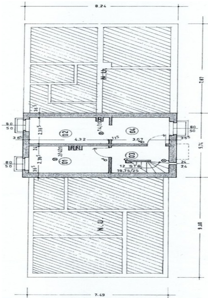
KELLERGEHOSS GRUNDRISS
