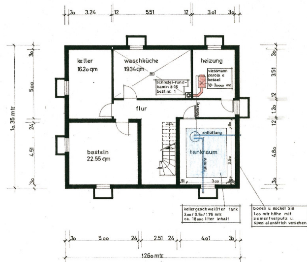
kellergeschoss
