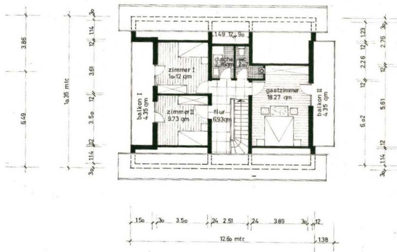
dachgeschoss
