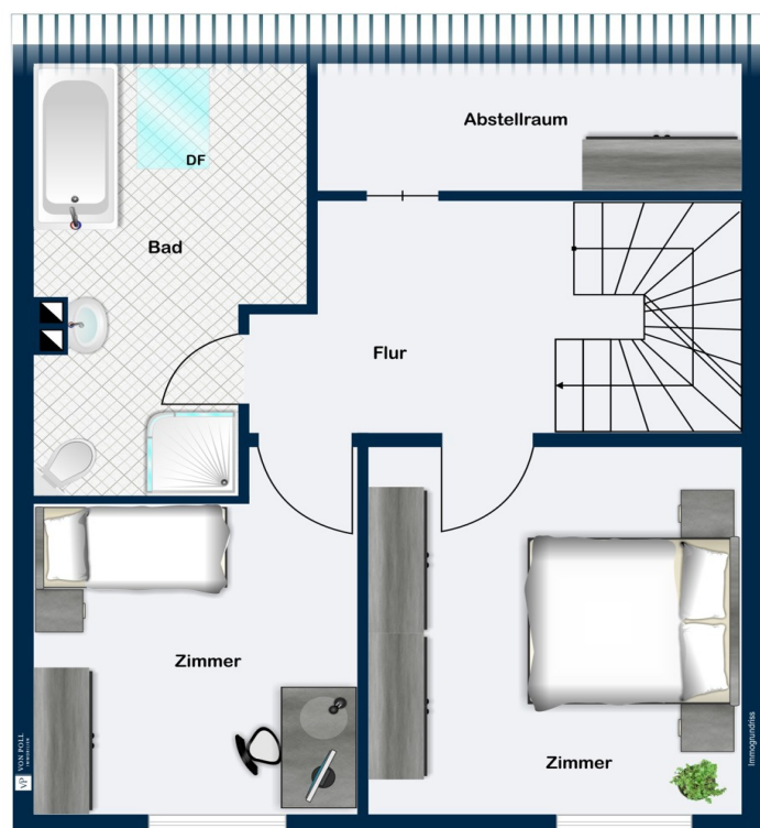
Obergeschoss
