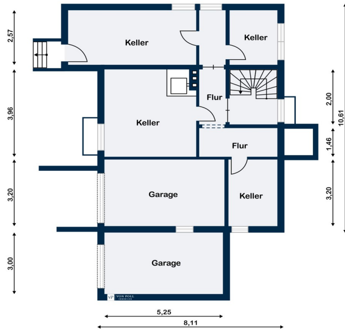
Kellergeschoss
