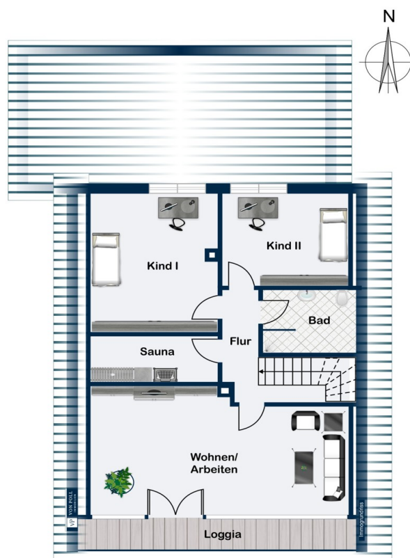
Dachgeschoss
