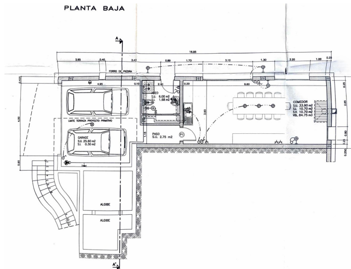
PLANTA SEMISOTANO
