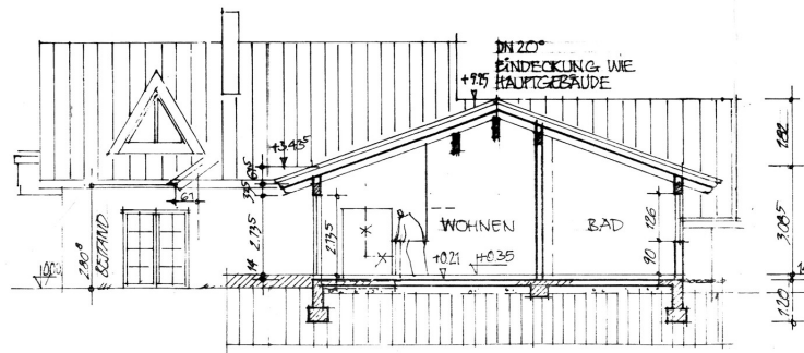
SCHNITT A-A
