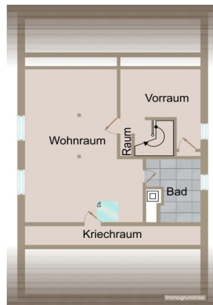
Dachgeschoss
