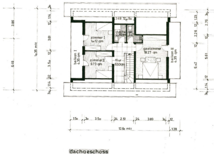
dachgeschoss
