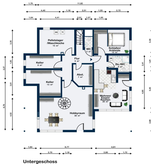
Untergeschoss
