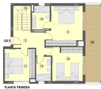
PLANTA PRIMERA
