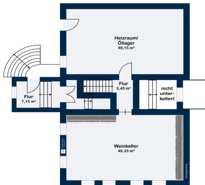
Untergeschoss
